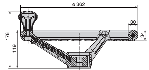
Con pomello - With knob
