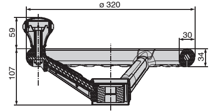
Con pomello - With knob
